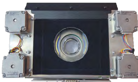
モジュール① CMYと補正フラグ、固定カラーホイール、2つの回転ゴボホイール
