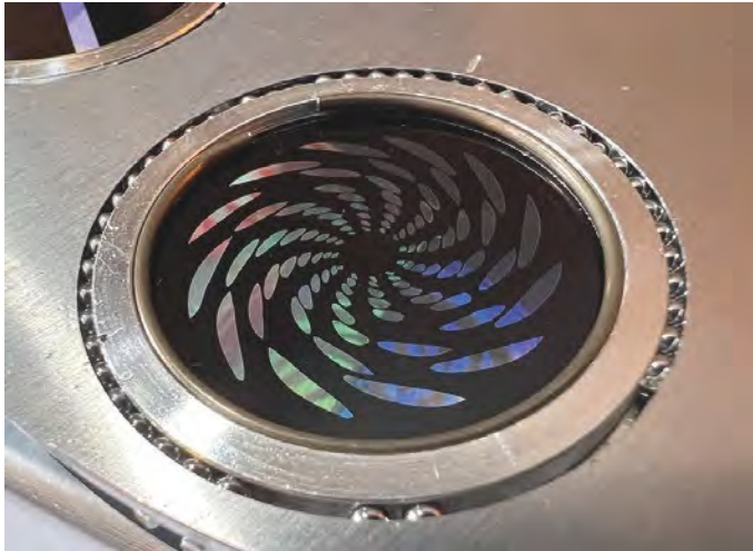
円形3方向または直線5方向プリズムで使用されているゴボ
